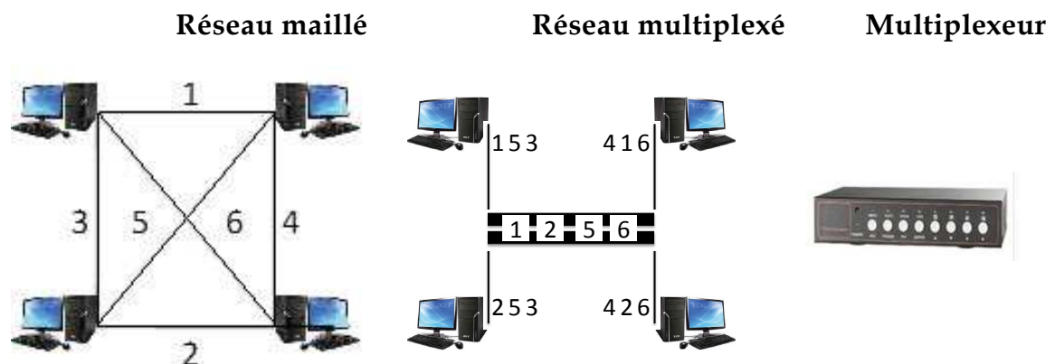
Schéma n° 17 : Le multiplexage
