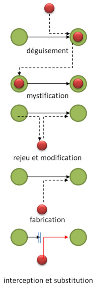
Schéma n° 82 : Modes opératoires combinés pour une attaque avancée
