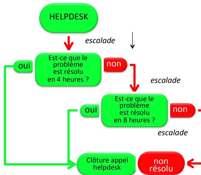
Schéma n° 89 : Circuit du traitement de l'incident de sécurité jusqu'à sa résolution
