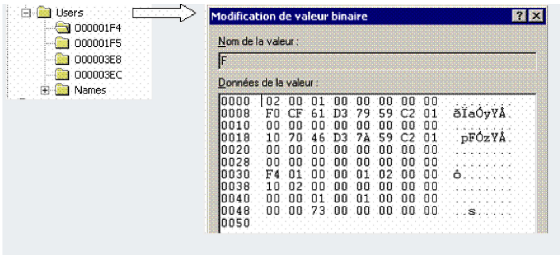
Schéma n° 62 : Espace de stockage des login /mots de passe sur un serveur
