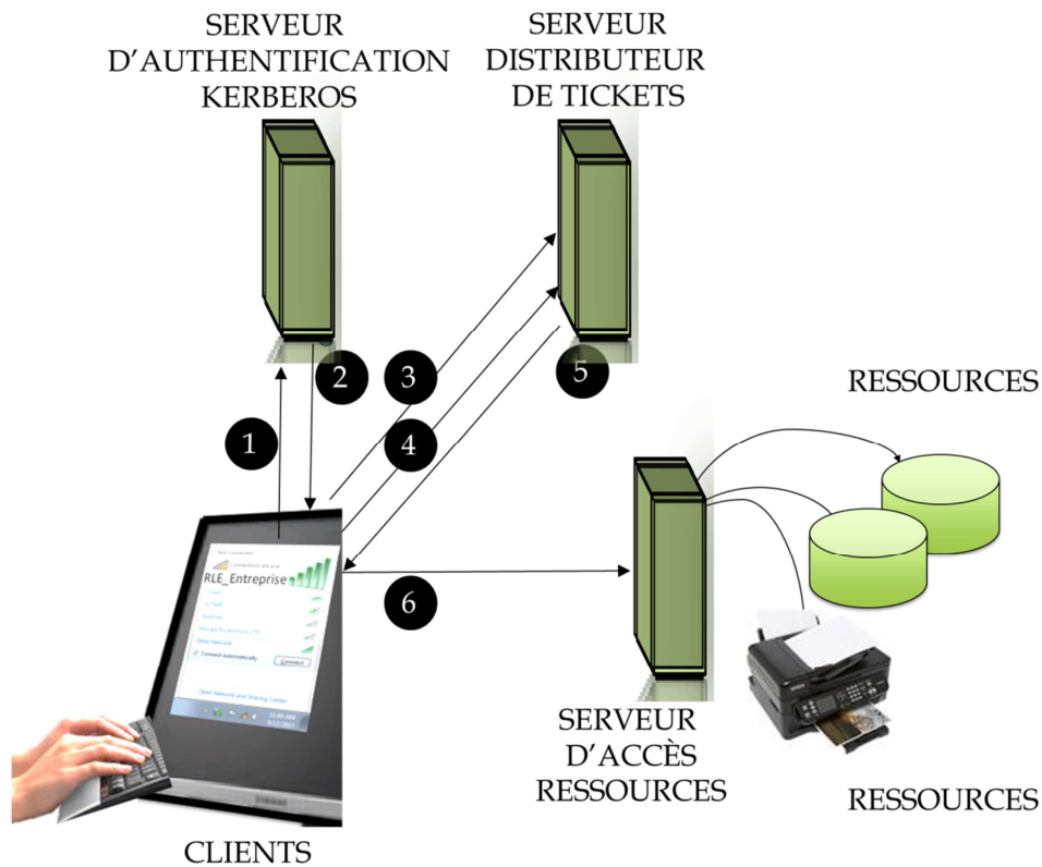
Schéma n° 68 : Processus d'authentification Kerberos en vue de l'obtention d'habilitation sur des ressources partagées
