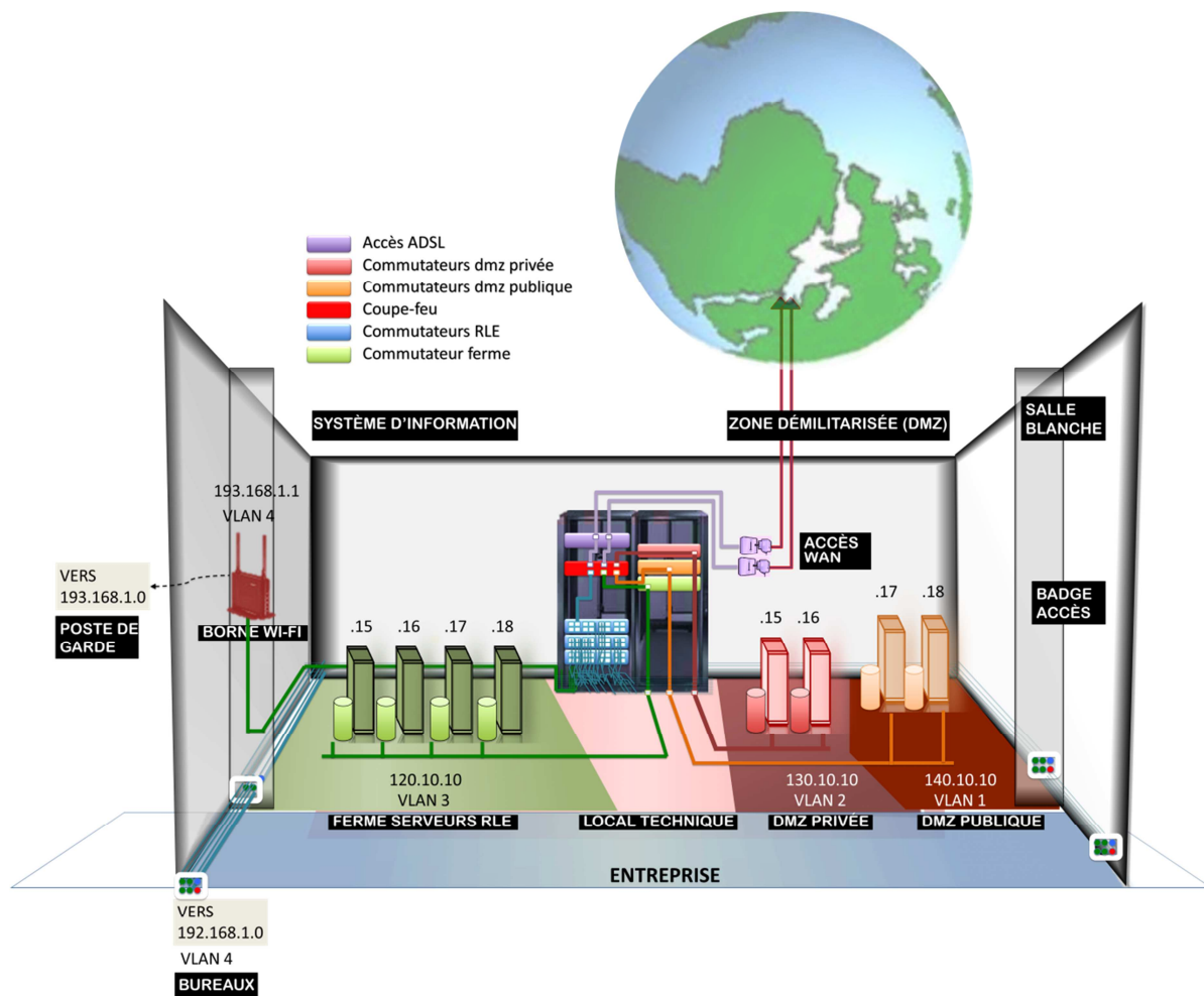
Schéma n° 56 : Architecture de sécurisation d'un système d'information
