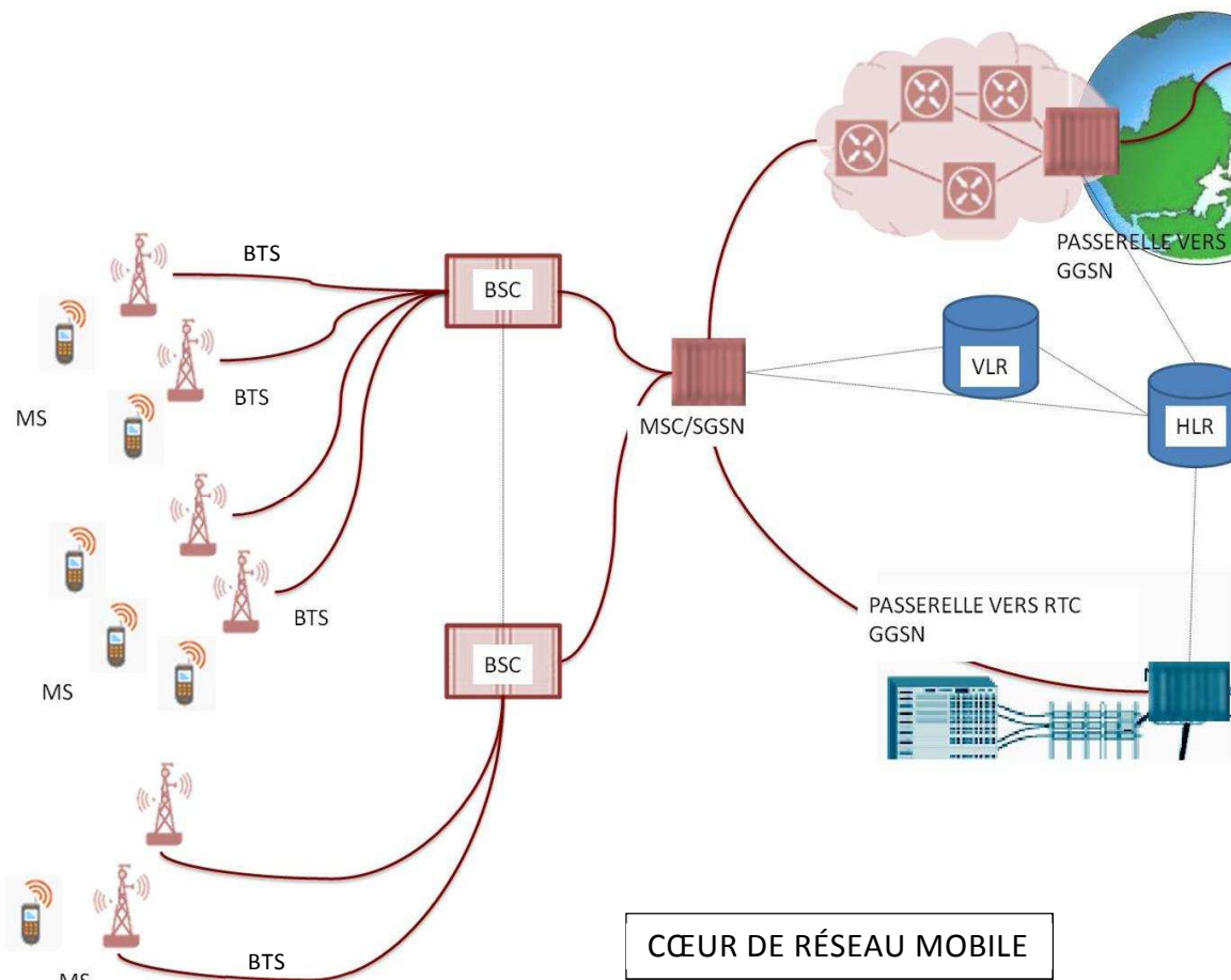
Schéma n° 24 : L'exemple d'un réseau 3G
